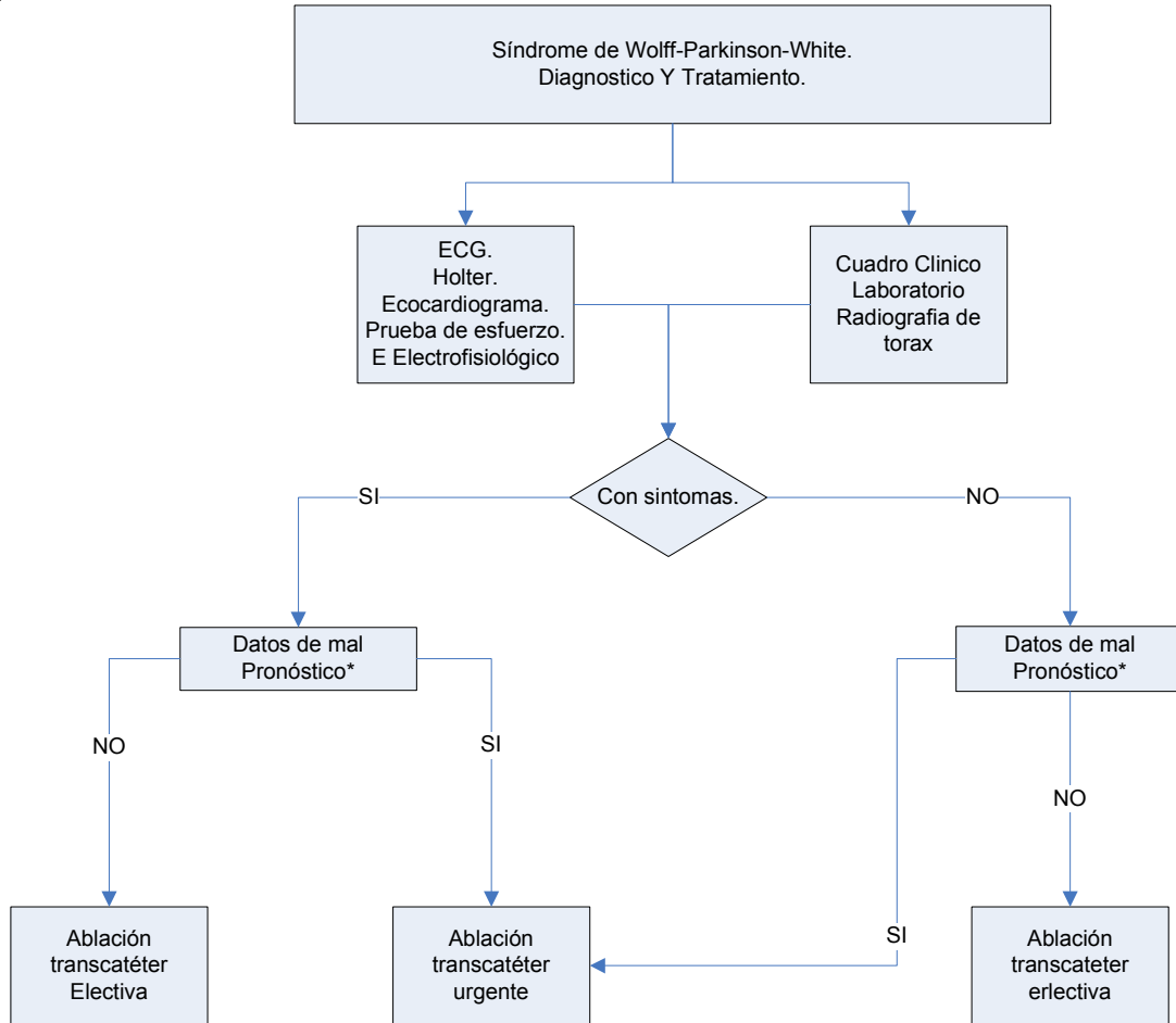
Algoritmo 1
